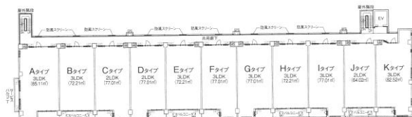
3～4階平面図
